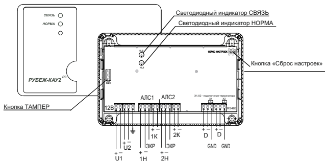
Рисунок 1 – Внешний вид контроллера
